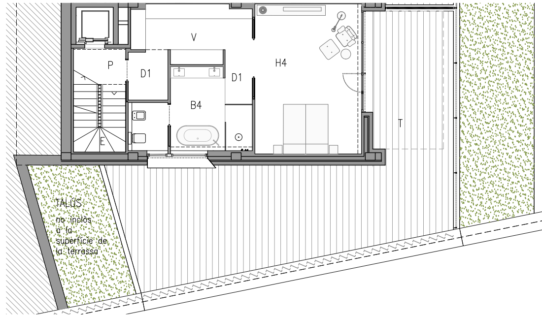
PLANTA BAIXA
