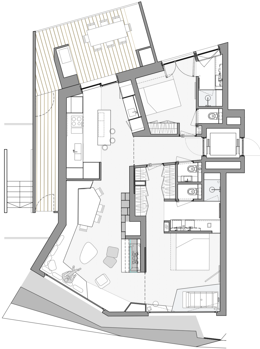
Planta segona / Second floor
