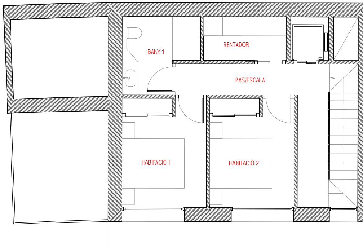
PLANTA PRIMERA
