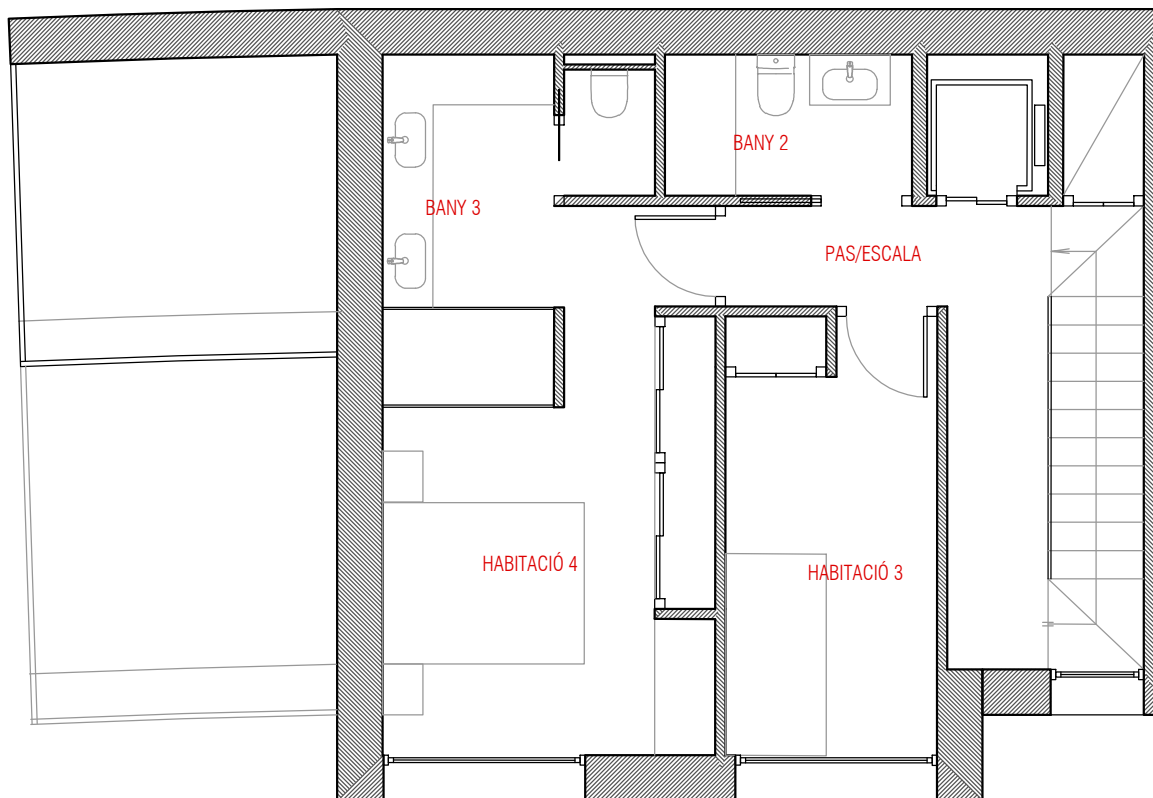
PLANTA SEGONA
