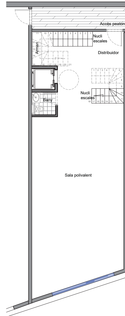
PLANTA -1
