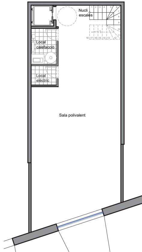
PLANTA -3
