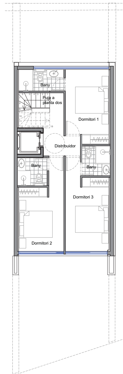
PLANTA PRIMERA
