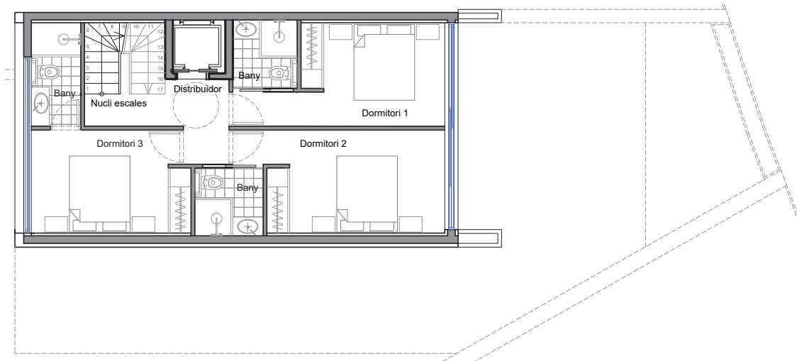
PLANTA PRIMERA
