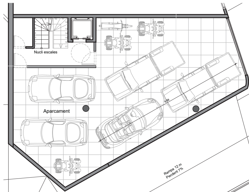
PLANTA -2
