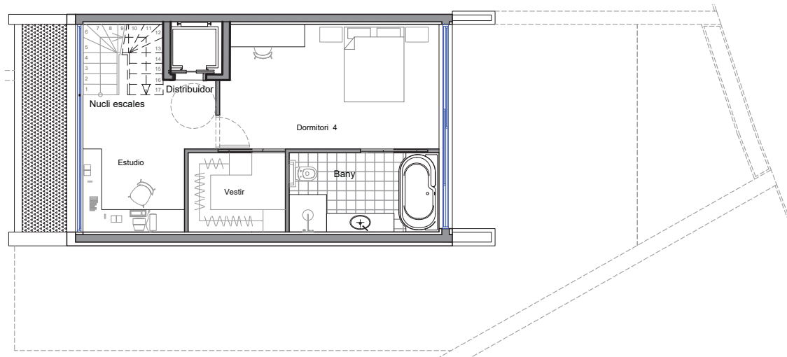
PLANTA SEGONA
